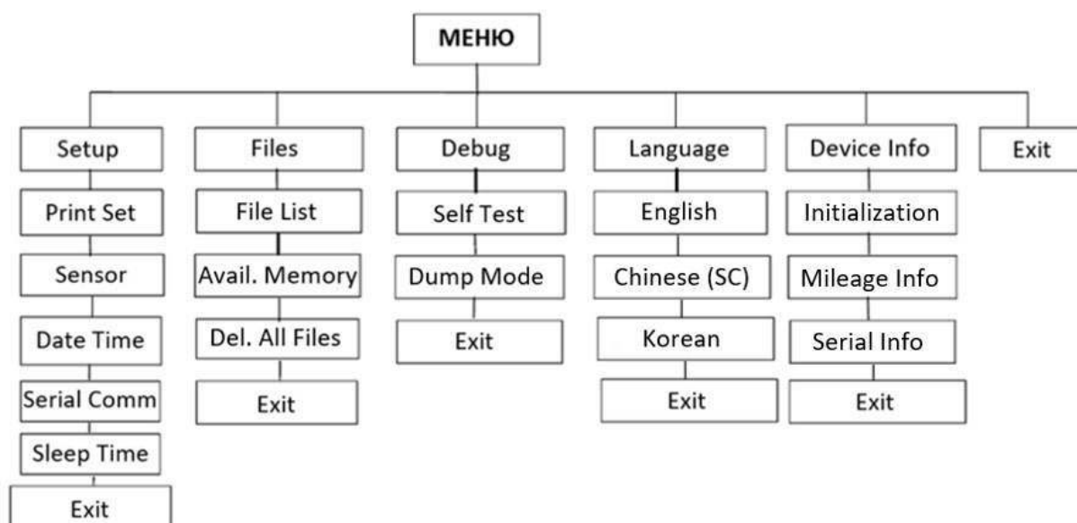
Рисунок 8. Структура меню принтера
